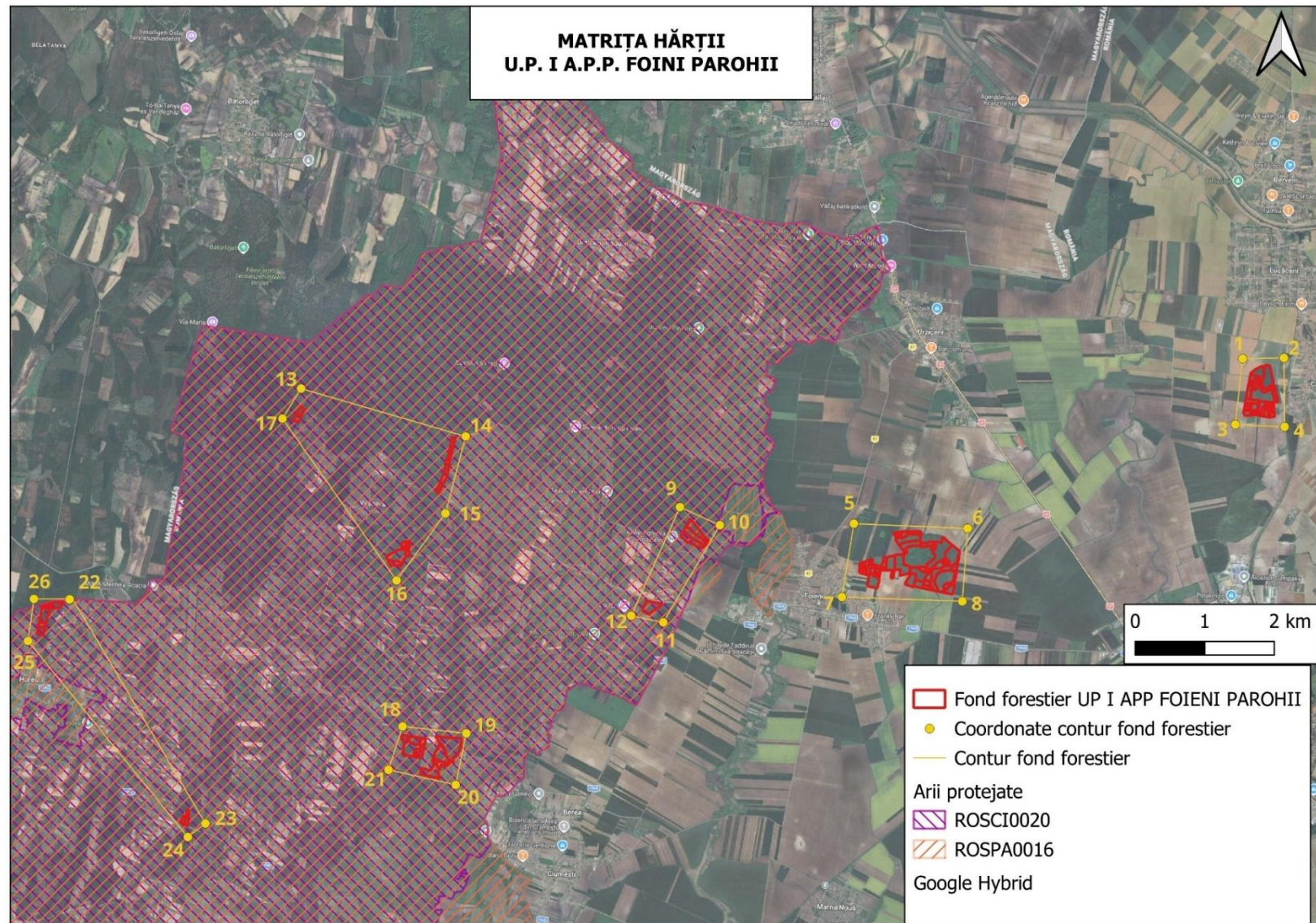
Fig. A.2.2 Conturul coordonatelor „Stereo 70” al punctelor ce încadrează suprafața inclusă în fondul forestier organizat în U.P. I A.P.P. Foieni-Parohii
